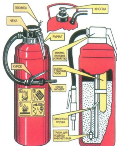
Порошковый огнетушитель
