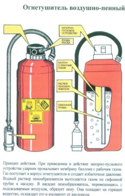
Приведение в действие воздушно-пенного огнетушителя
